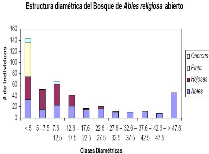
Figura 25. Estructura diamétrica del bosque de Abies religiosa abierto
