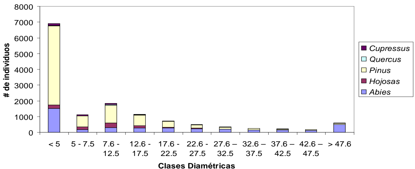
Figura 24. Estructura diamétrica de los bosques de la cuenca del Río Magdalena, D.F.
