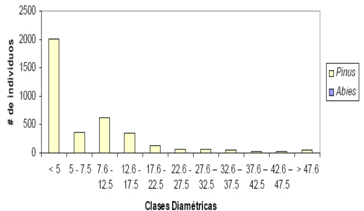
Figura 29. Estructura diamétrica del bosque de Pinus hartwegii cerrado
