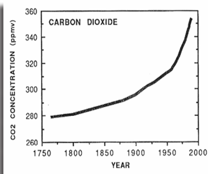
Figura 4. Incremento en la concentración de CO 2 en la atmósfera desde la época preindustrial al presente. (IPCC, 2007)
