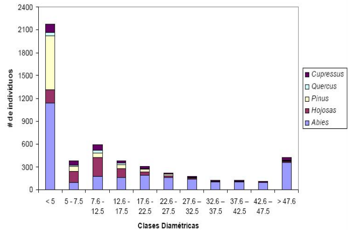
Figura 26. Estructura diamétrica del bosque de Abies religiosa cerrado
