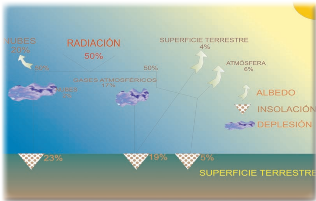
Figura 2. Equilibrio Radiactivo (Garcia, 1989)
