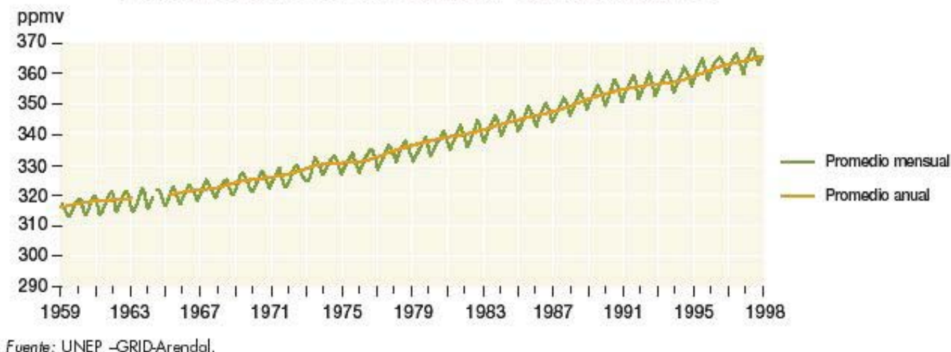
Figura 5. Concentración de CO 2 en la atmósfera; Estación Mauna Loa (sanfern.iies.es, 2006)
