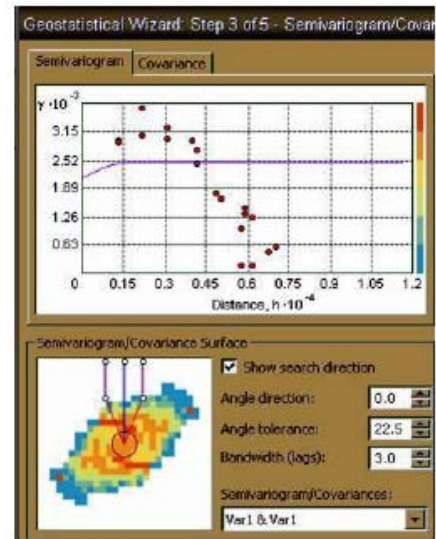
Figura 32. Semivariograma de los valores reales del Contenido de Carbono
