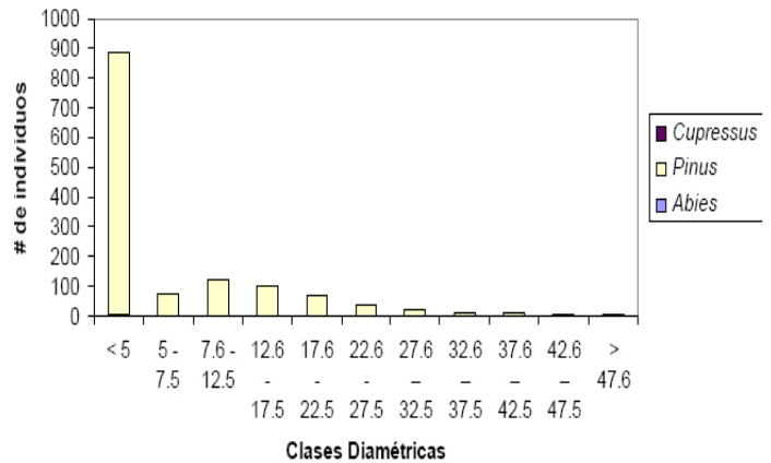
Figura 28. Estructura diamétrica del bosque de Pinus hartwegii abierto
