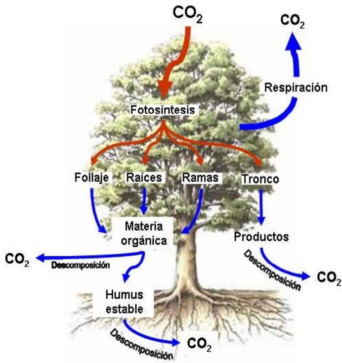
Figura 7. Flujos y almacenes de carbono en un ecosistema forestal (Fragoso, 2003).
