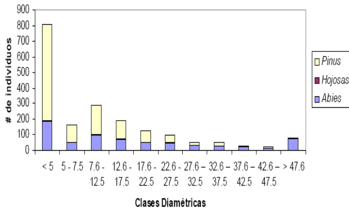
27. Estructura diamétrica del bosque de Abies - Pinus cerrado
