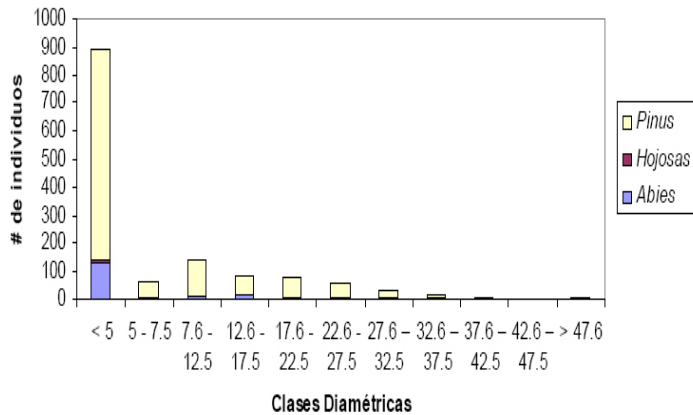
Figura 30. Estructura diamétrica del bosque de Pinus-Abies cerrado
