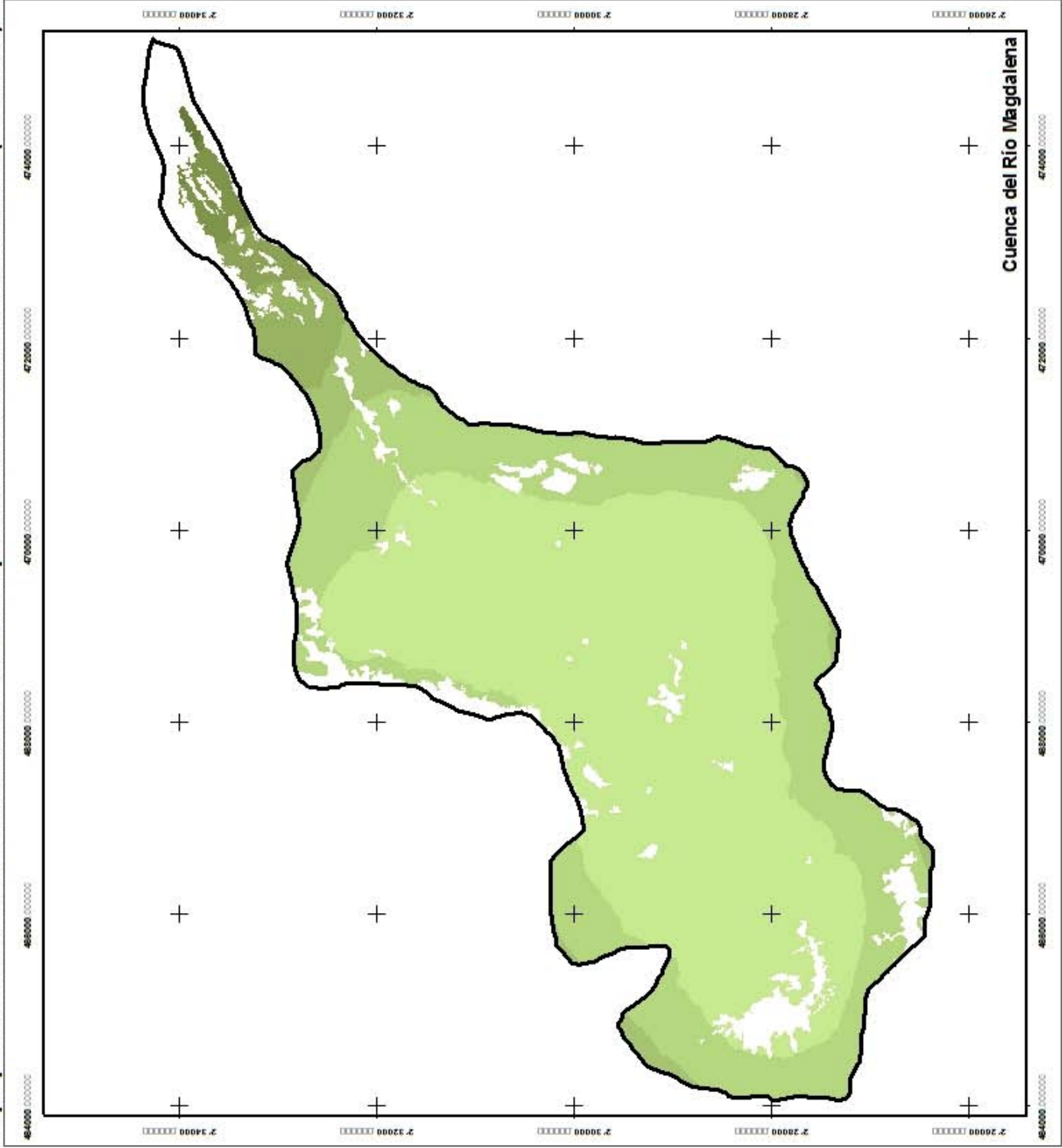
Figura 42. Mapa predictivo de los errores estándar de la Interpolación del Contenido de Carbono Promedio
