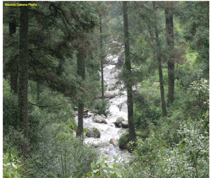
Figura 11. Bosque de Abies religiosa de la cuenca del Río Magdalena
