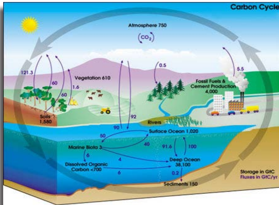
Figura 6. Ciclo de Carbono (es.wikipedia.org/wiki/Ciclo_del_carbono, 2006)
