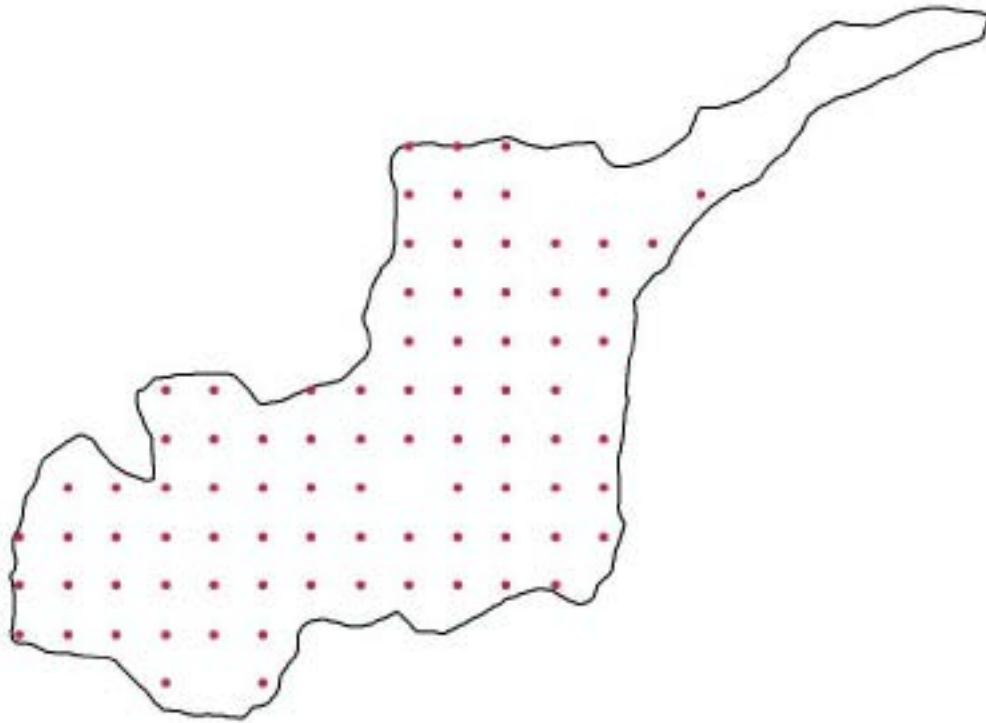
Figura 14. Red cuadrangular de puntos obtenidas del muestreo sistemático simple para la zona.
