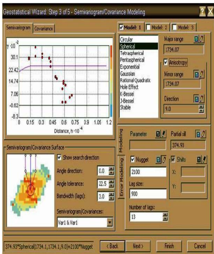
Figura 33. Modelo de semivariograma para el Contenido de Carbono Real
