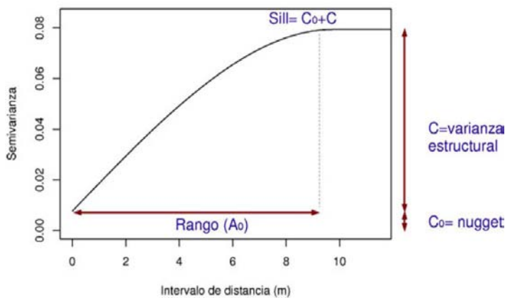
Figura 17. Parámetros de la estructura de un semivariograma (Gallardo, 2006)
