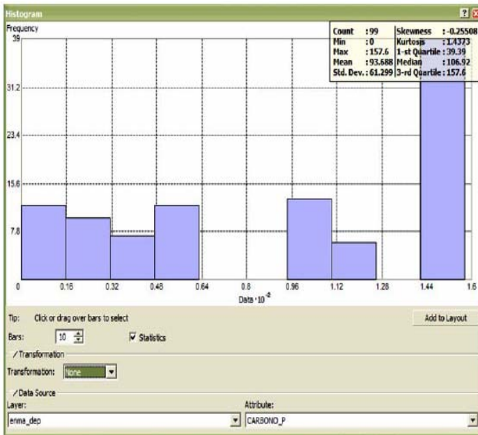
Figura 37. Estadísticos básicos de la distribución de la muestra (promedios)
