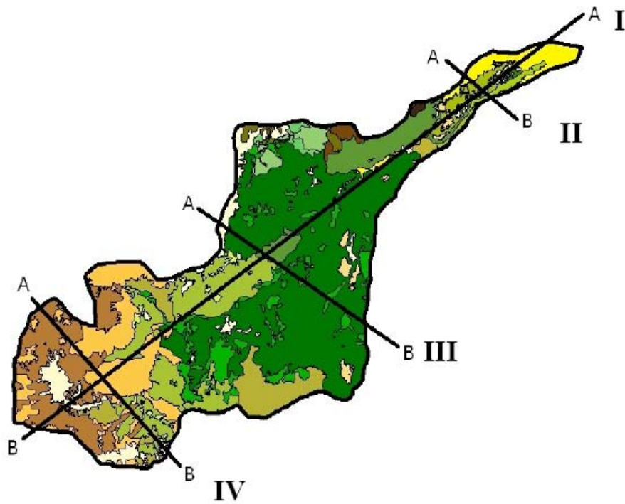
Figura 19. Mapas de Vegetación y Uso de Suelo con los cortes que dan origen a los perfiles
