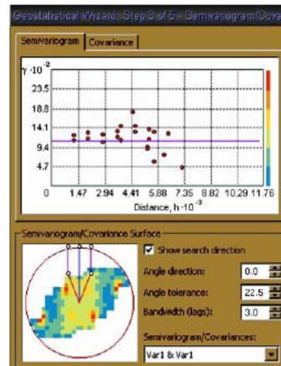
Figura 38. Semivariograma de los datos promedio del Contenido de Carbono
