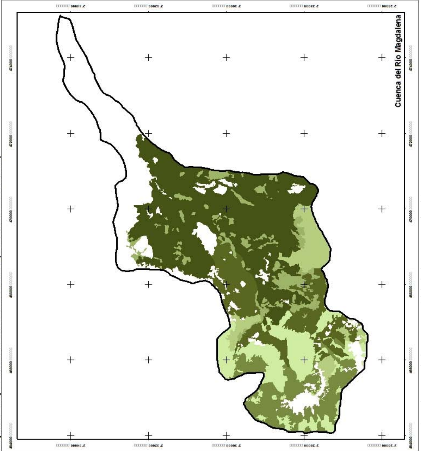
Figura 44. Mapa de Captura Potencial de Carbono (Escenario a 25 años).
