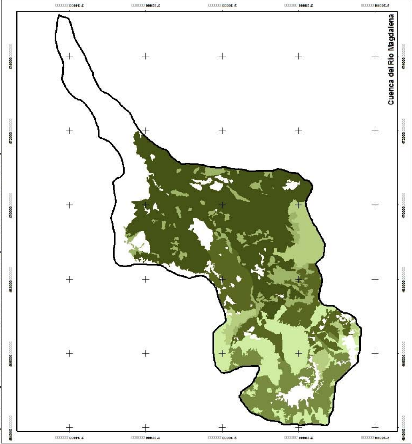
Figura 45. Mapa de Captura Potencial de Carbono (Escenario a 50 años).
