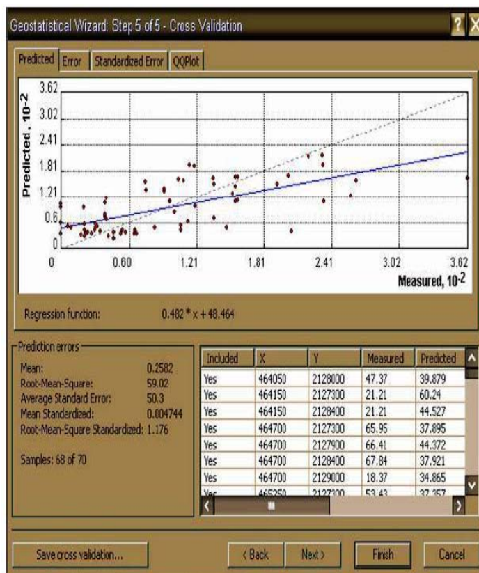
Figura 34. Validación cruzada y estadísticos de los errores de la predicción
