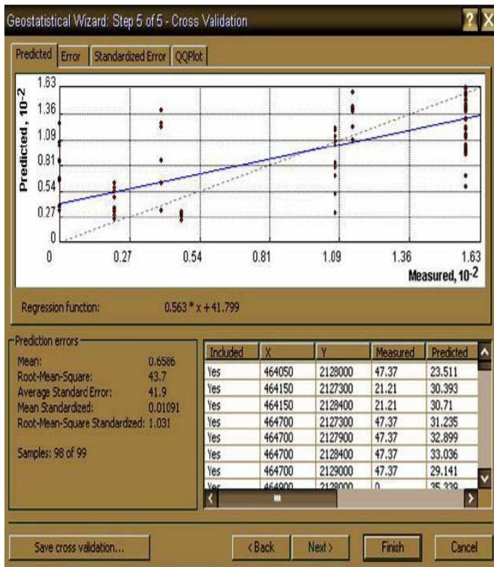
Figura 40. Validación cruzada y estadísticos de los errores de la predicción
