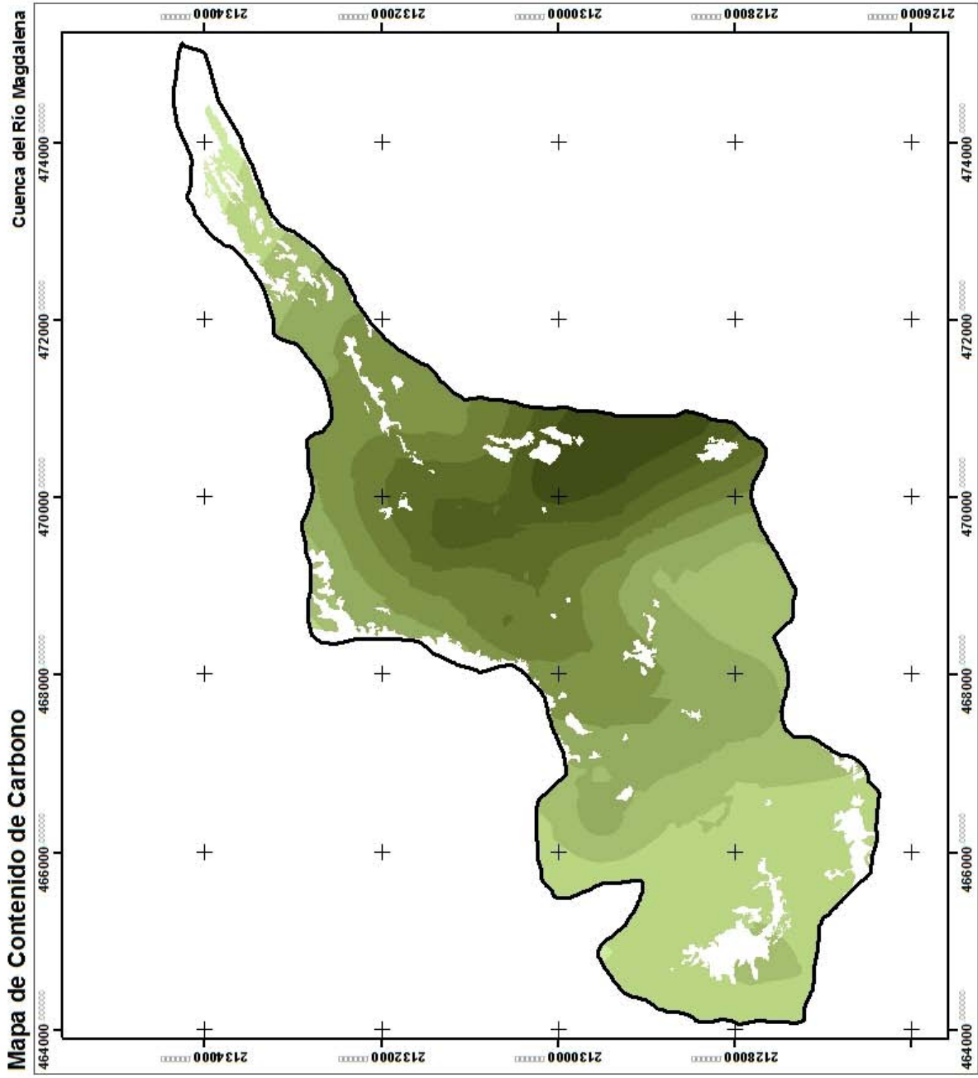
Figura 35. Mapa de Contenido de Carbono
