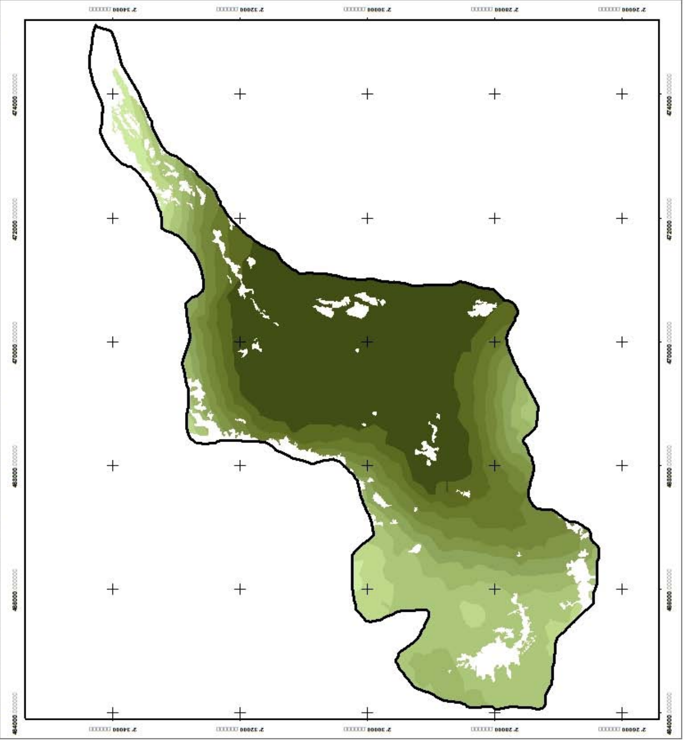
Figura 41. Mapa de Contenido de Carbono Promedio
