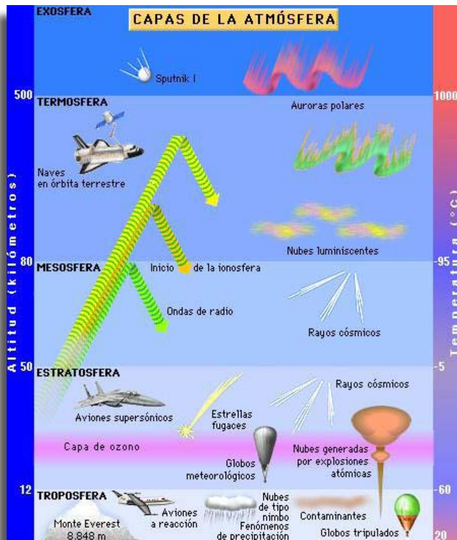
Figura 1. Ilustración de las capas que componen la atmósfera (recursos.cnice.mec.es)
