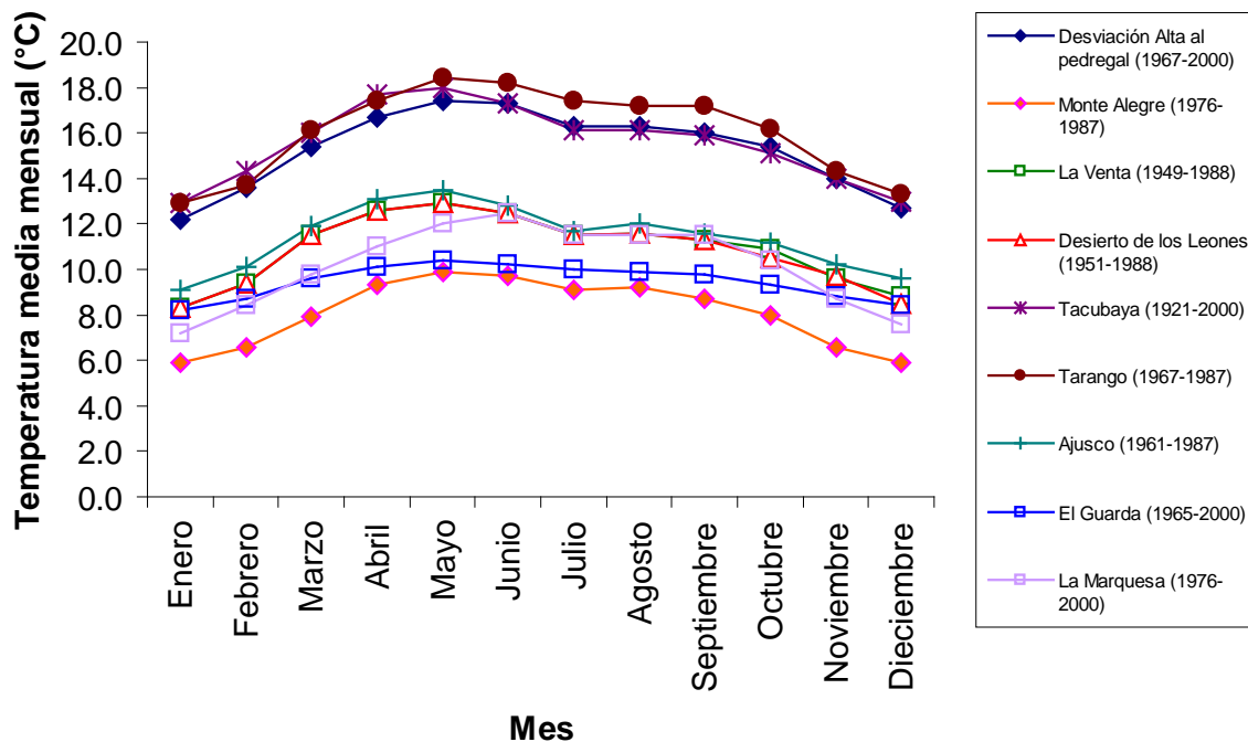
Figura 9. Temperaturas medias mensuales comprendidas en la zona de estudio (INEGI, 2005; ver anexo cartográfico)
