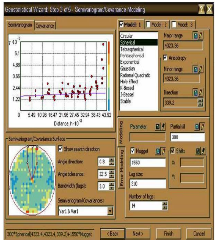
Figura 39. Modelo de semivariograma para el Contenido de Carbono Promedio
