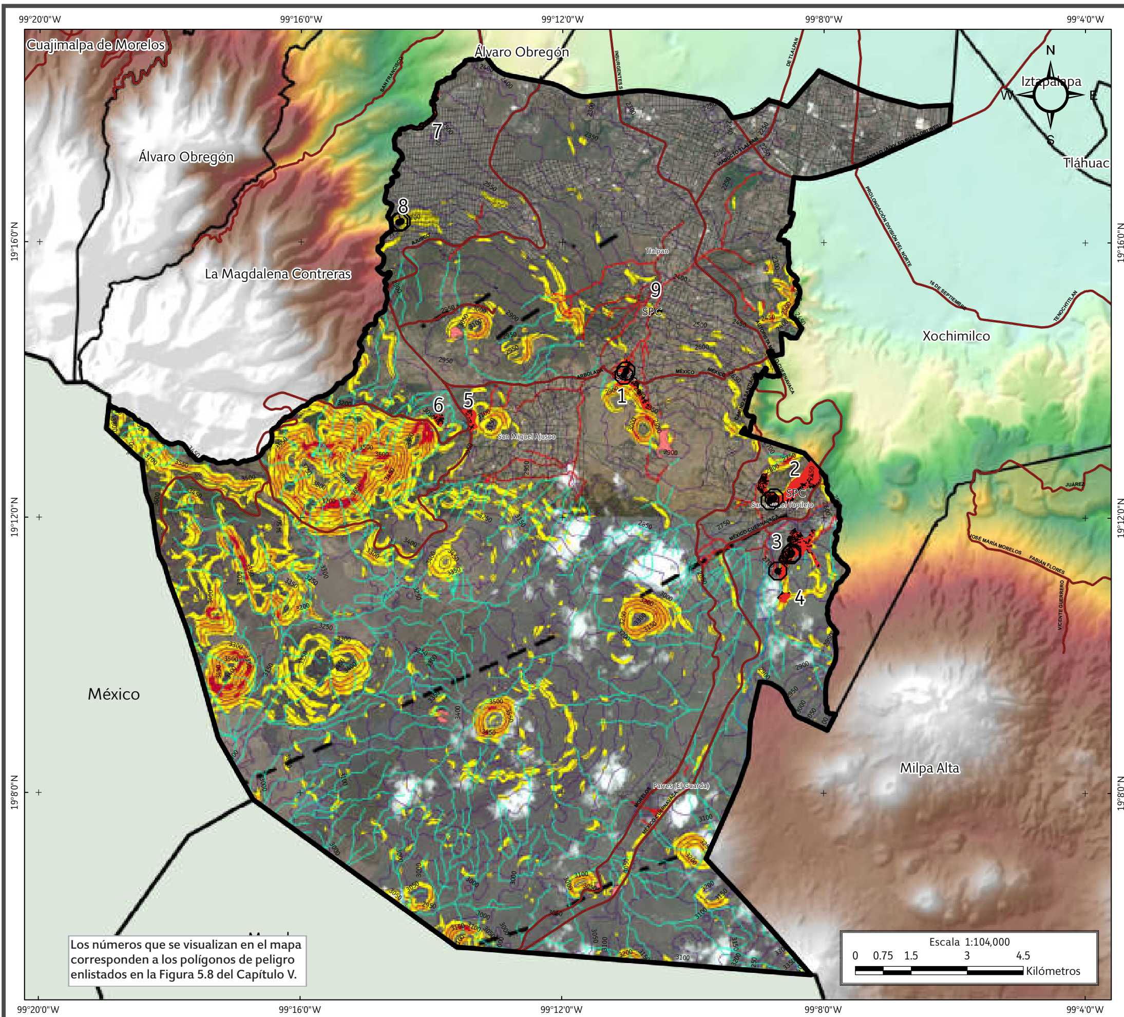
Mapa XXII. Riesgos por fenómenos de remoción en masa.
