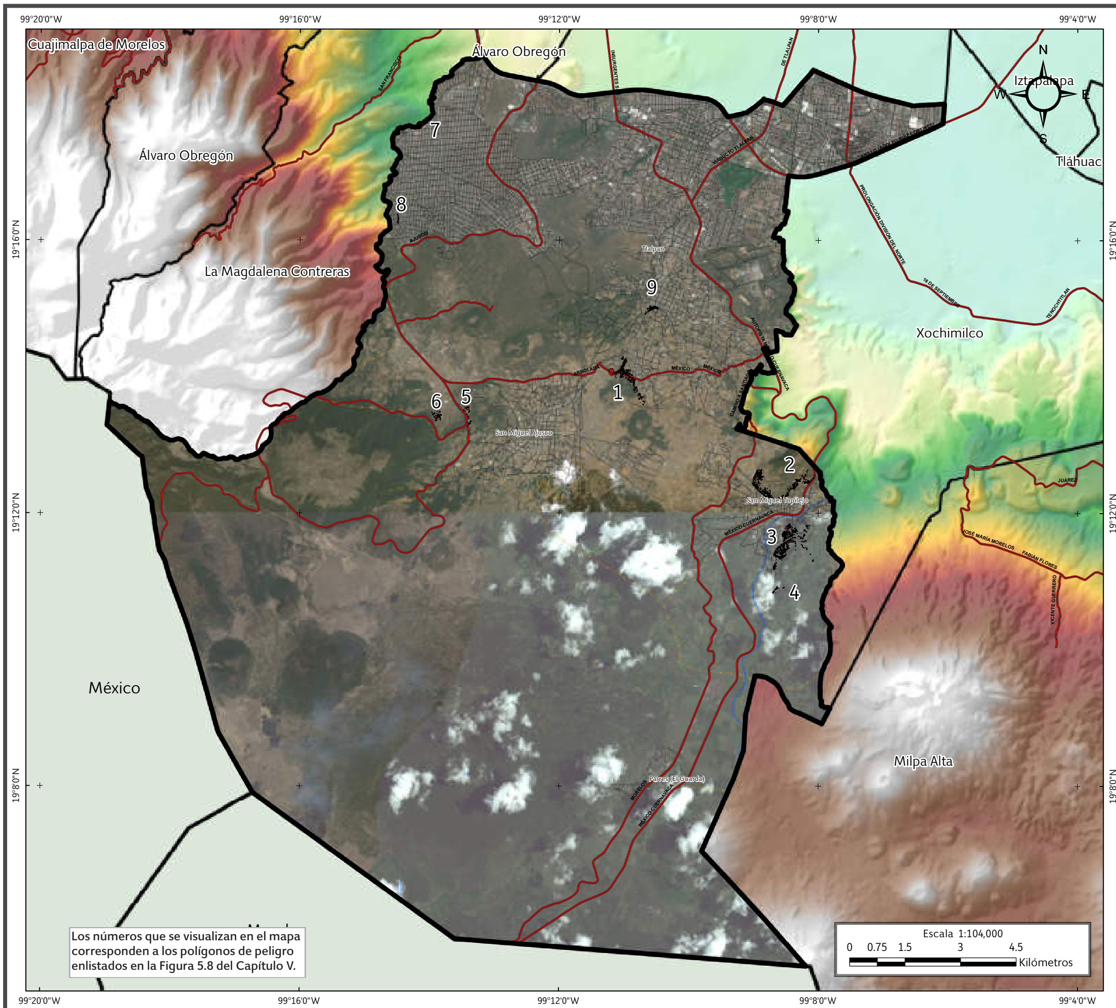
Mapa XXI. Vulnerabilidad por fenómenos de remoción en masa.
